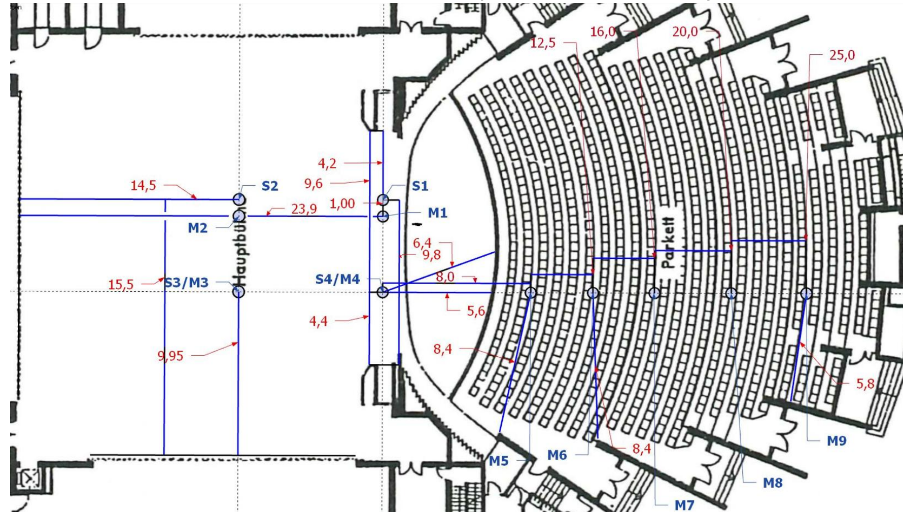
Grundriss Opernhaus mit Messpositionen
